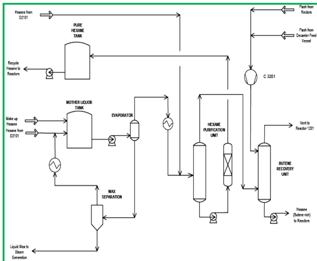
شکل ۴-۰: طرح کلی پلای اتیلن سنگین
