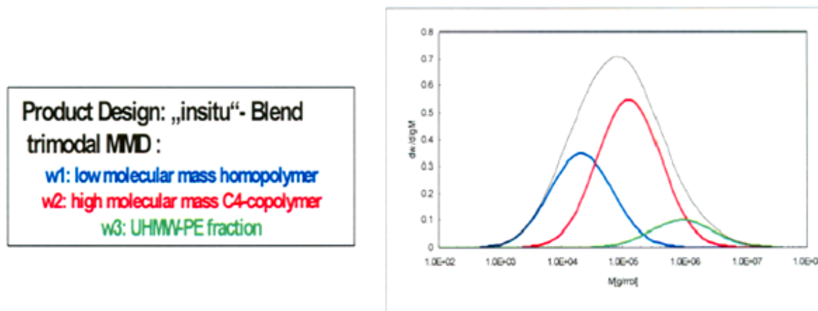
شکل ۲-۰: نمودار زیر توزیع وزن مولکولی هر کدام از اجزاء مخلوط داخل راکتور در فرآیند Hostalen ACP.
