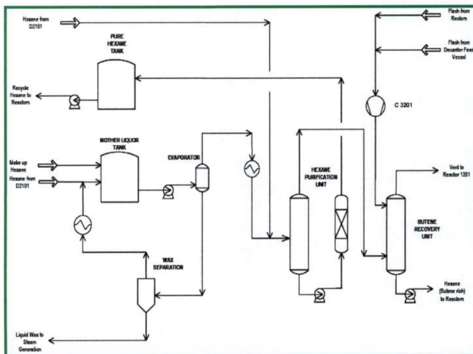
شکل ۴-۰: طرح کلی پلی اتیلن سنگین
