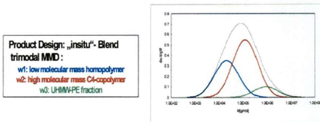
شکل ۲-۰: نمودار توزیع وزن مولکولی هر کدام از اجزاء مخلوط داخل راکتور در فرآیند Hostalen ACP
