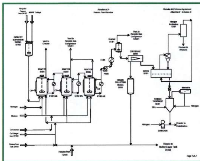
شکل ۴-۰: طرح کلی پلی اتیلن سنگین
