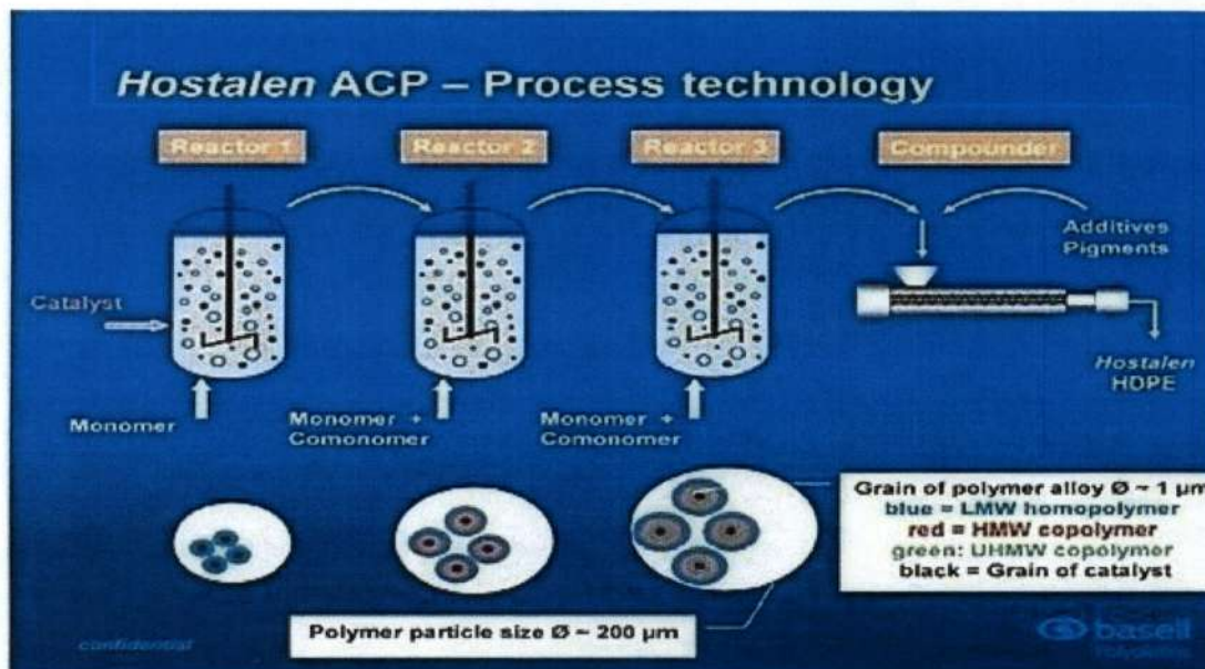
شکل ۱-۰: شمایی از فرآیند Hostalen ACP:
